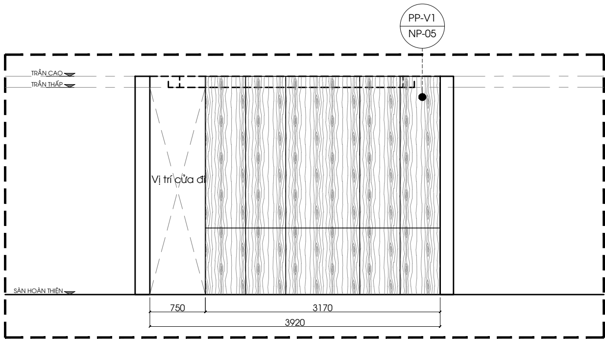
PN1 MẶT ĐỨNG 4 - 1:50 @ A3
