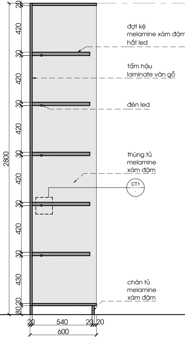
PN1-01- MẶT CẮT 3 1:20 @ A3
