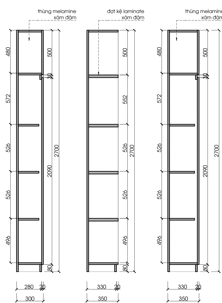
MẶT CẮT S-01 1:20 @A3
