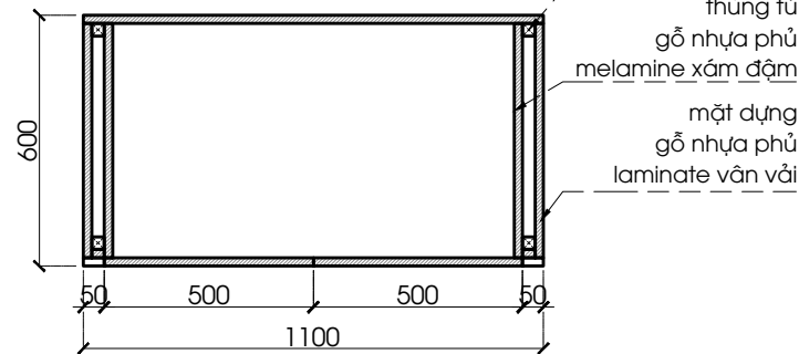
PN1-07 - MẶT CẮT NGANG 1:20 @ A3
