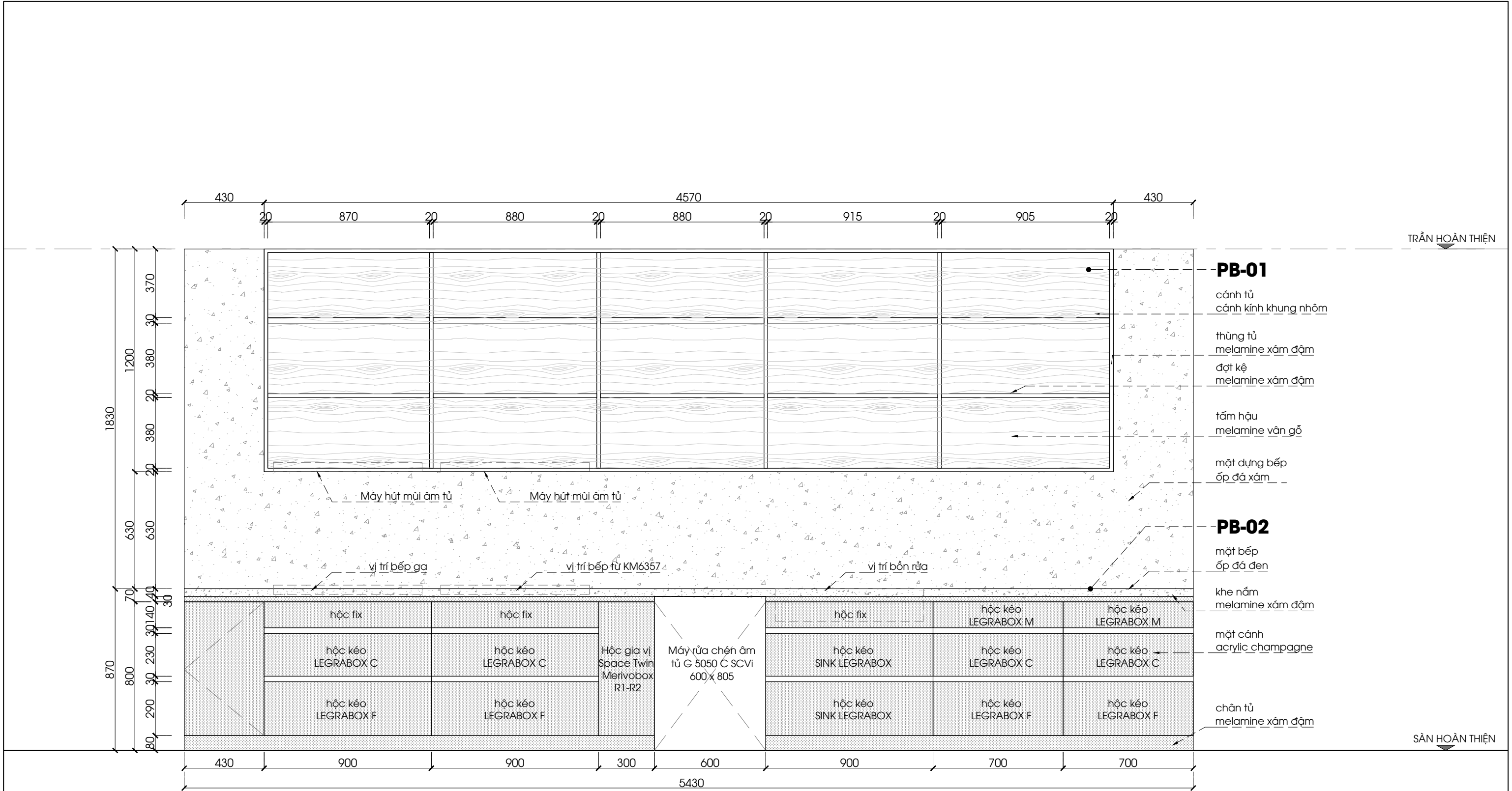
PB-01 & PB-02 - MẶT ĐỪNG - KHÔNG CẢNH
