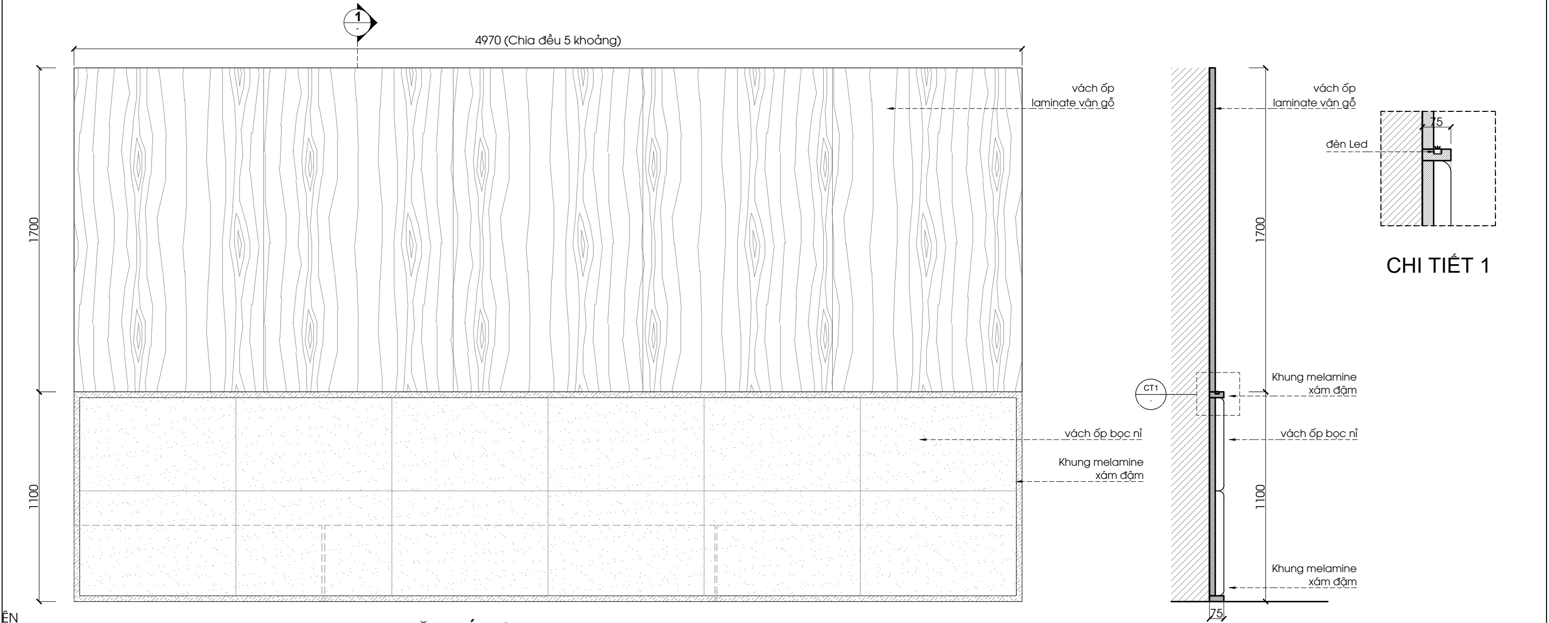
MẶT CẮT 1 1:20 @A3
