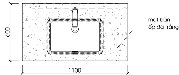
PN1-07 - MẶT BẰNG 1:20 @ A3
