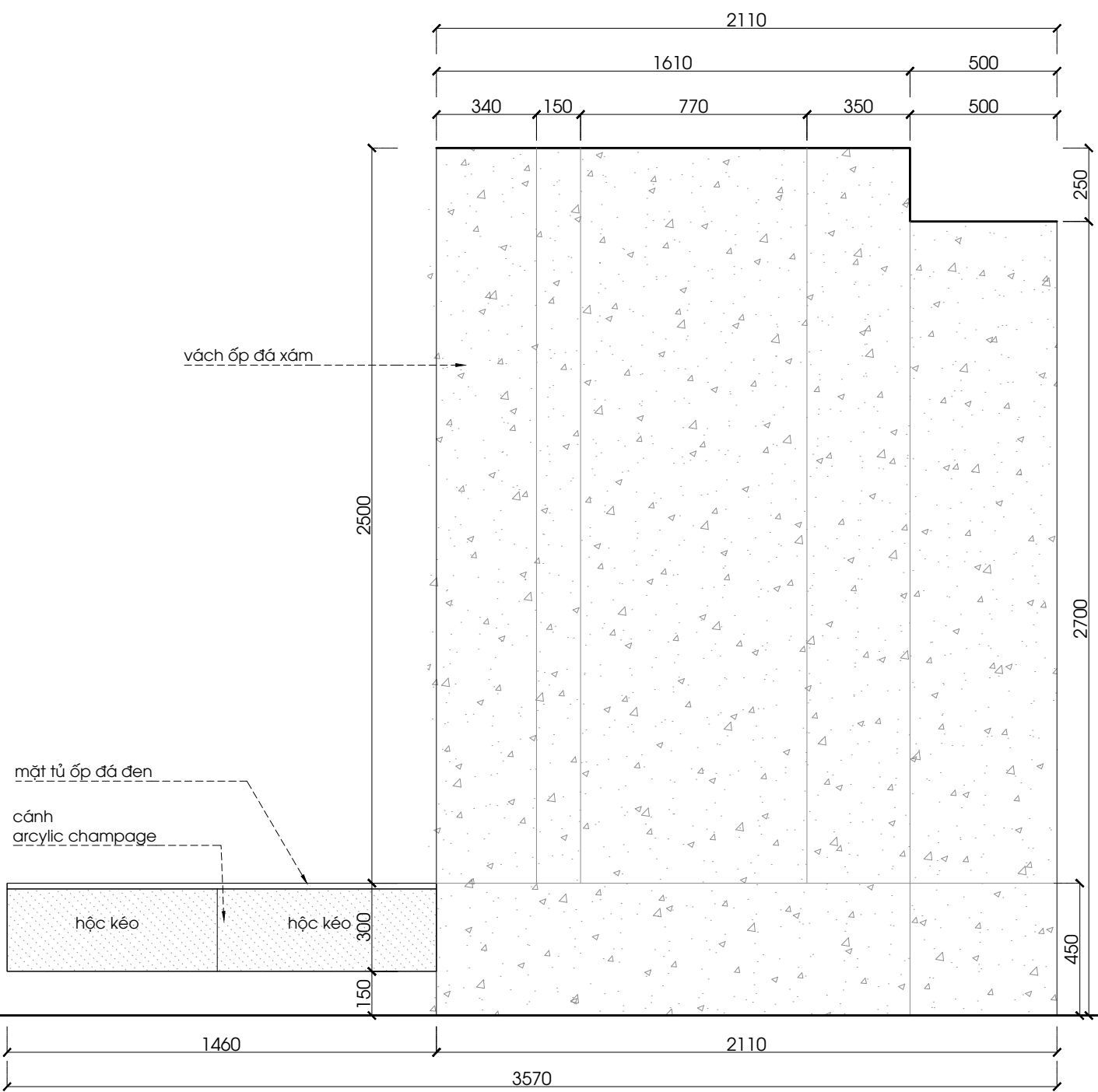
MẶT ĐỪNG 3 PK-01 1:20 @A3
