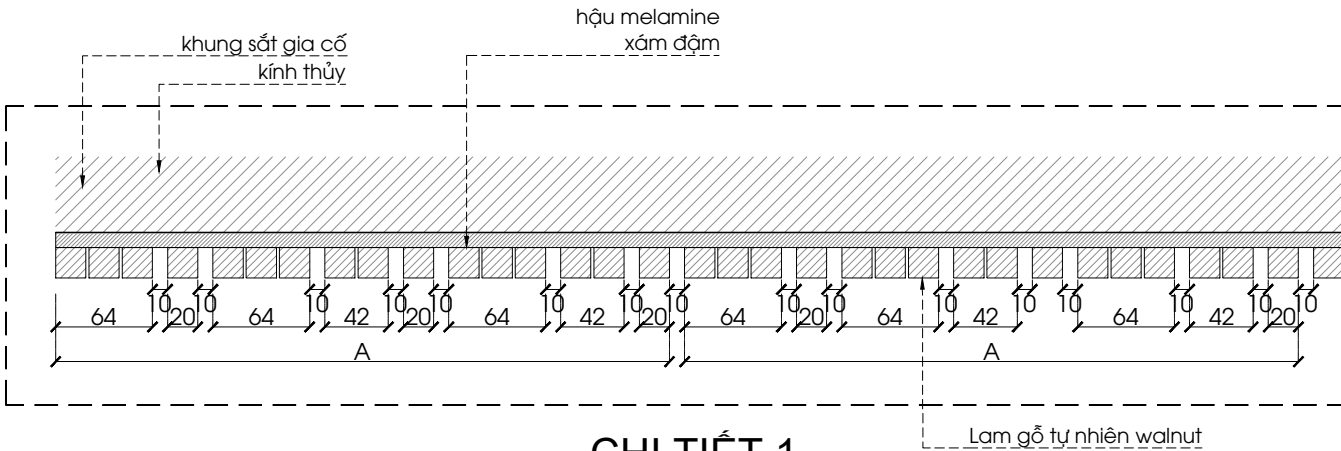
CHI TIẾT 1
