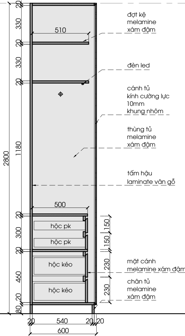
PN1-01- MẶT CẮT 2 1:20 @ A3
