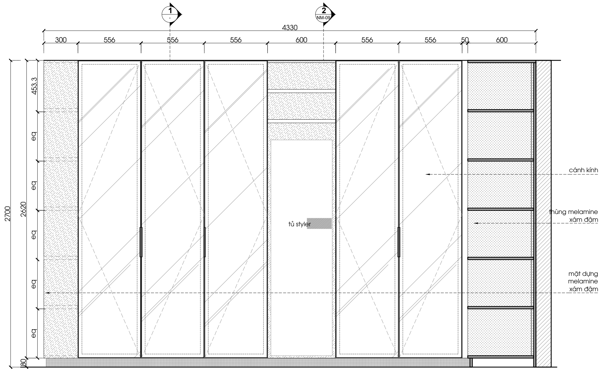
MẶT ĐỨNG PM-06 1:20 @A3
