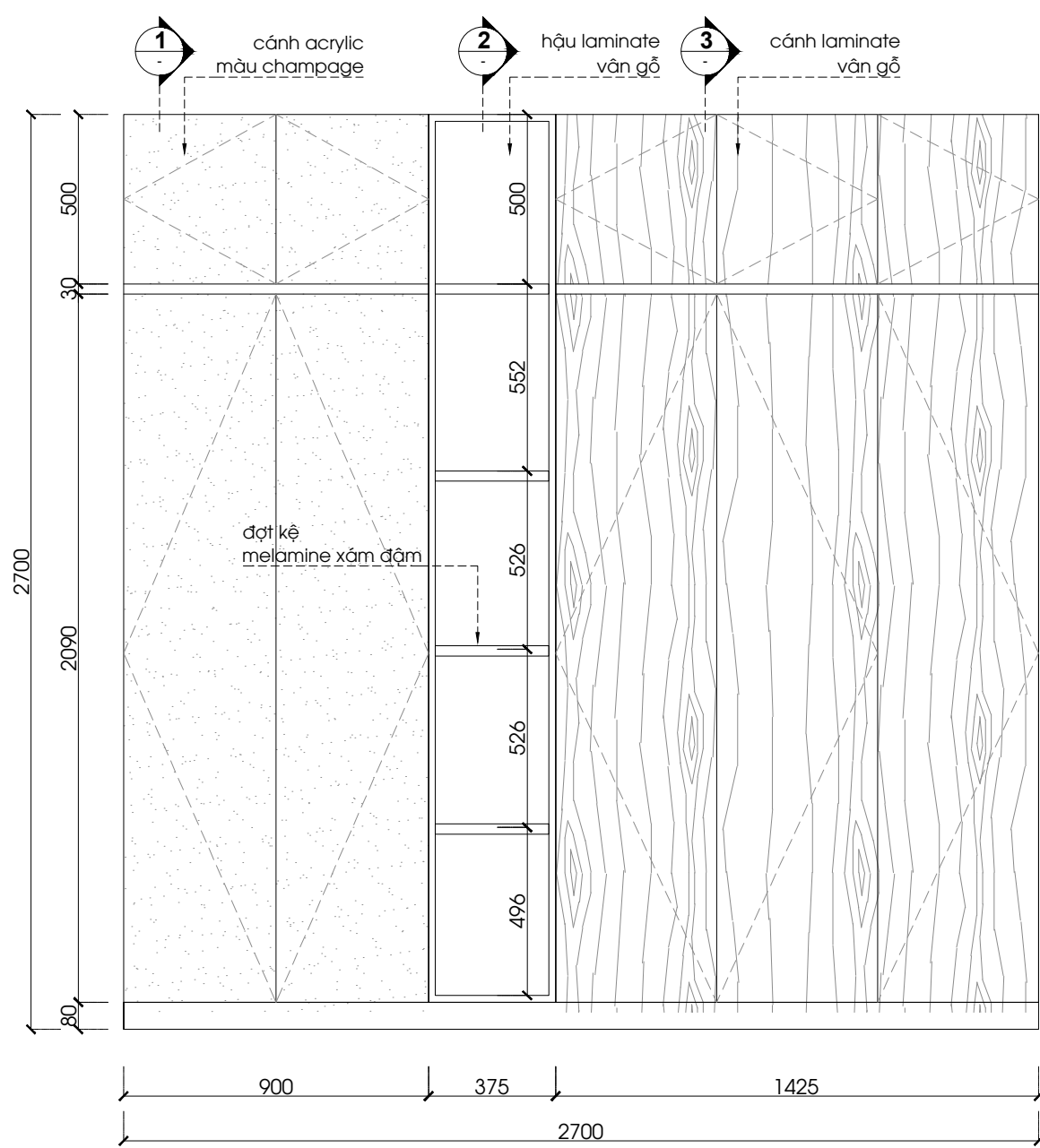
MẶT ĐỨNG S-01,02,03 1:20 @A3
