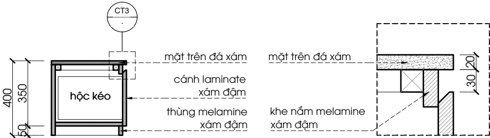
MẶT CẮT 2 1:20 @A3
