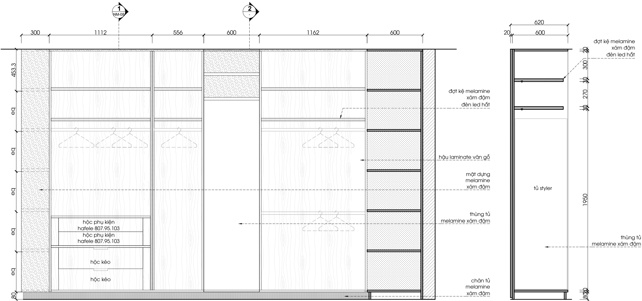
MẶT ĐỨNG THÙNG TỦ PM-06 1:20 @A3
