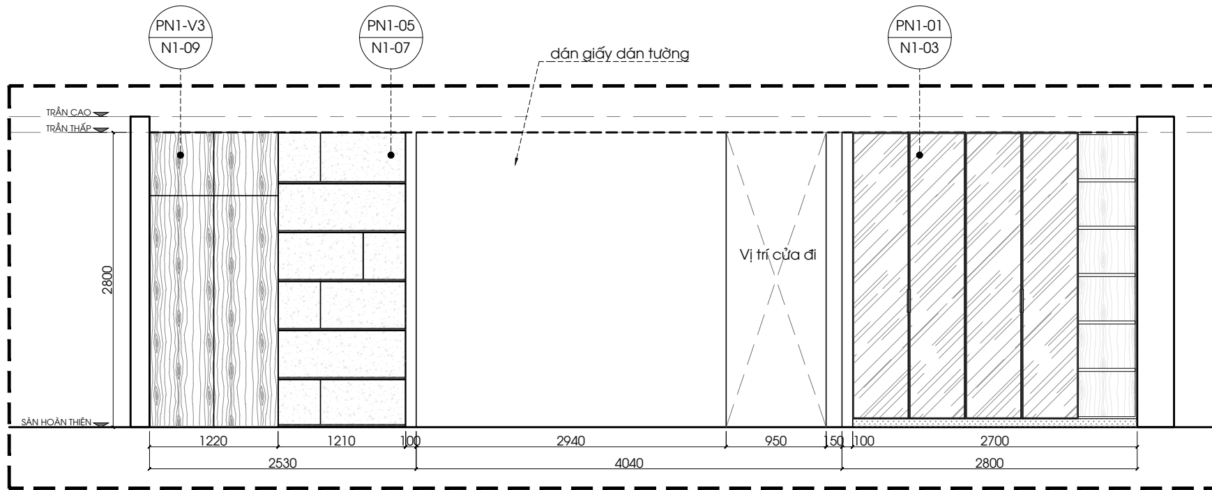
PN1 MẶT ĐỨNG 2
