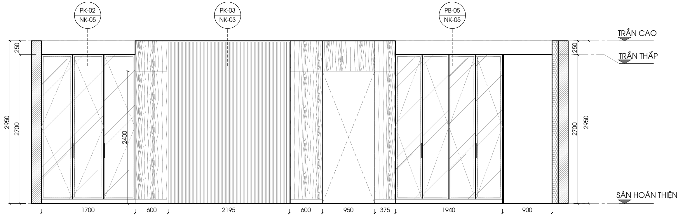
MẶT ĐỨNG 1 1:40 @A3
