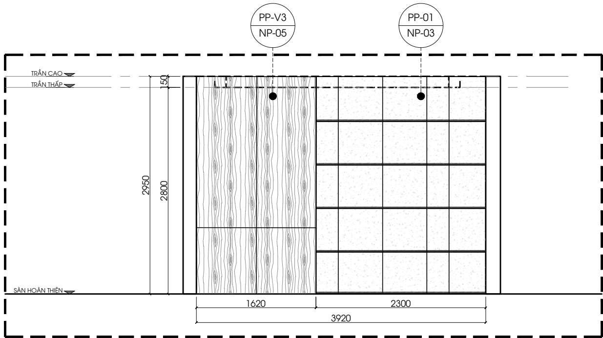
PN1 MẶT ĐỨNG 2 - 1:50 @ A3
