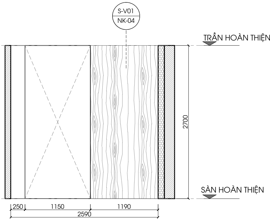
MẶT ĐỨNG 3 1:40 @A3
