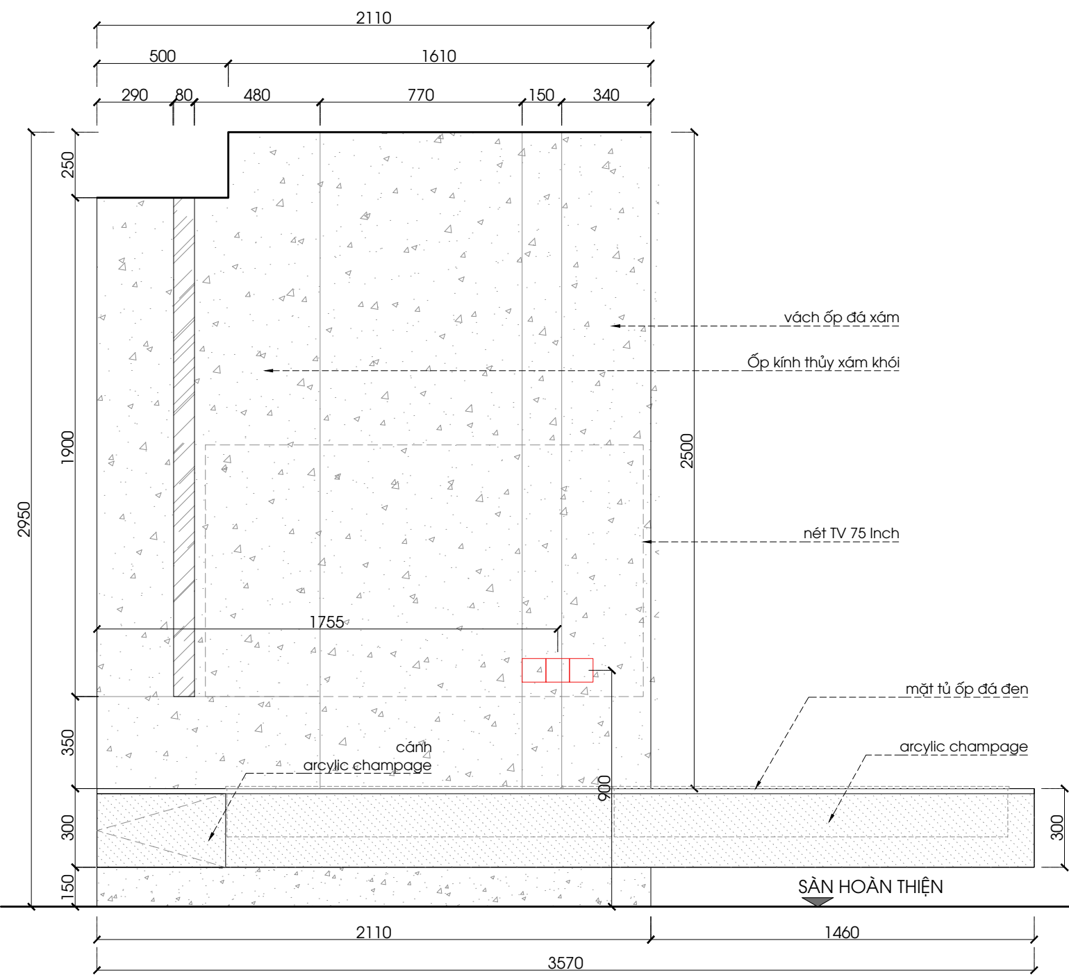
MẶT ĐỪNG 2 PK-01 1:20 @A3
