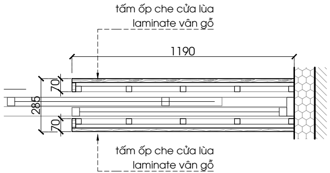
MẶT BẰNG S-V01 1:20 @A3
