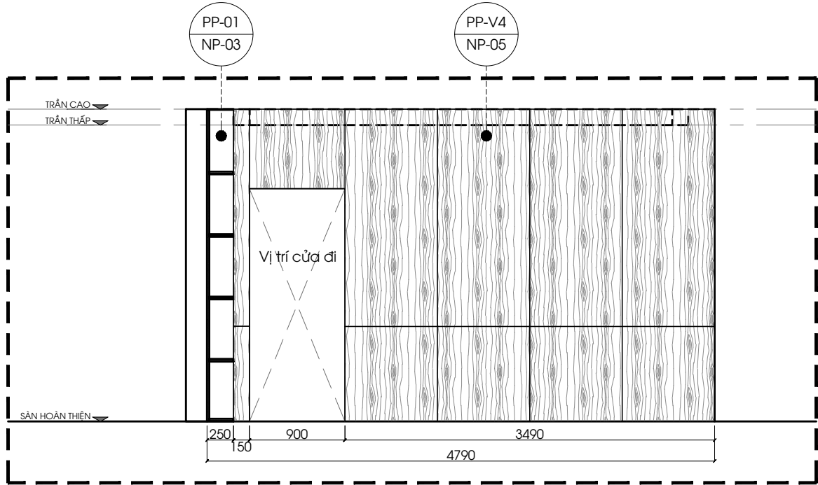
PN1 MẶT ĐỨNG 3 - 1:50 @ A3
