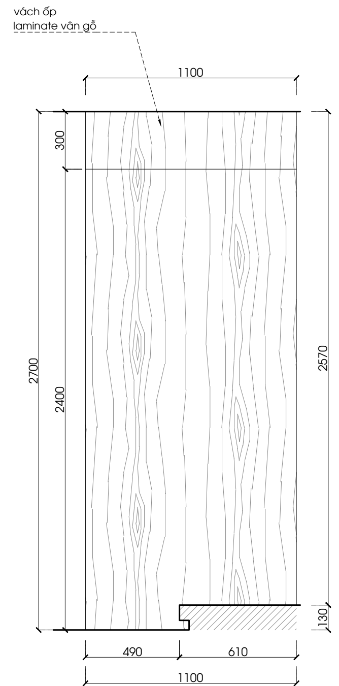
MẶT ĐÚNG PM-V8 1:20 @A3
