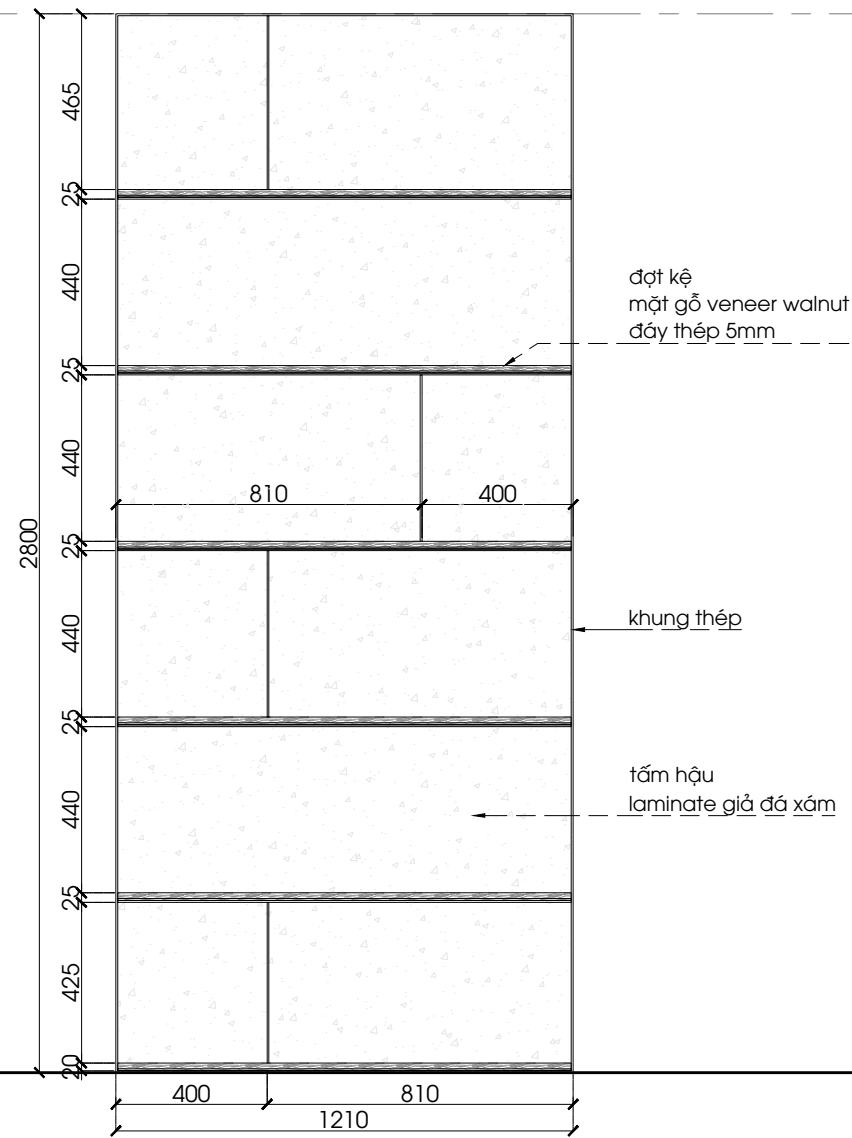
PN1-05 - MẶT ĐỨNG
