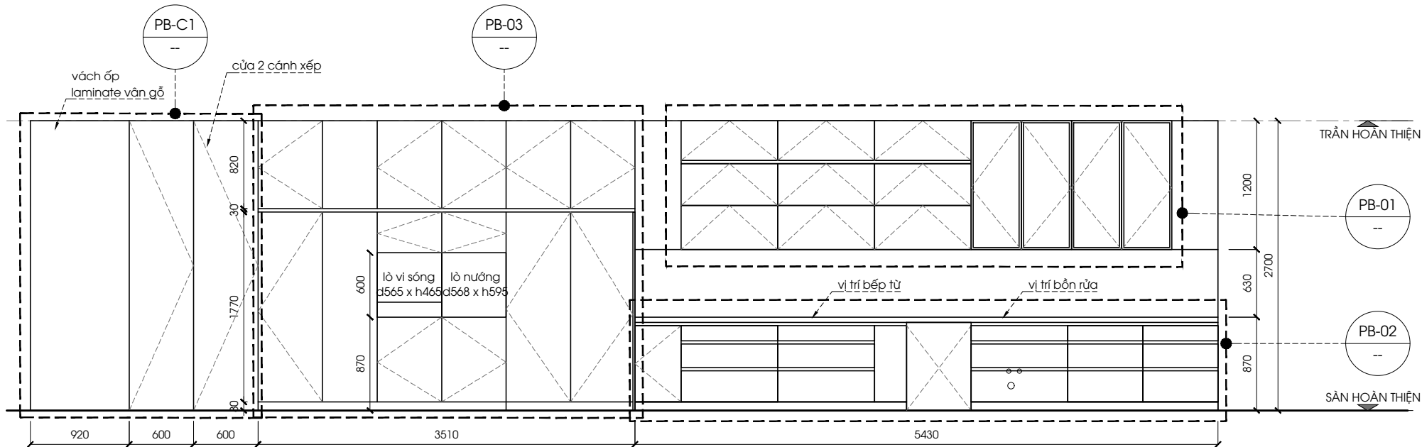
MẶT ĐỨNG HỆ TỦ BẾP
