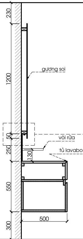
WC-01 MẶT CẮT 1
