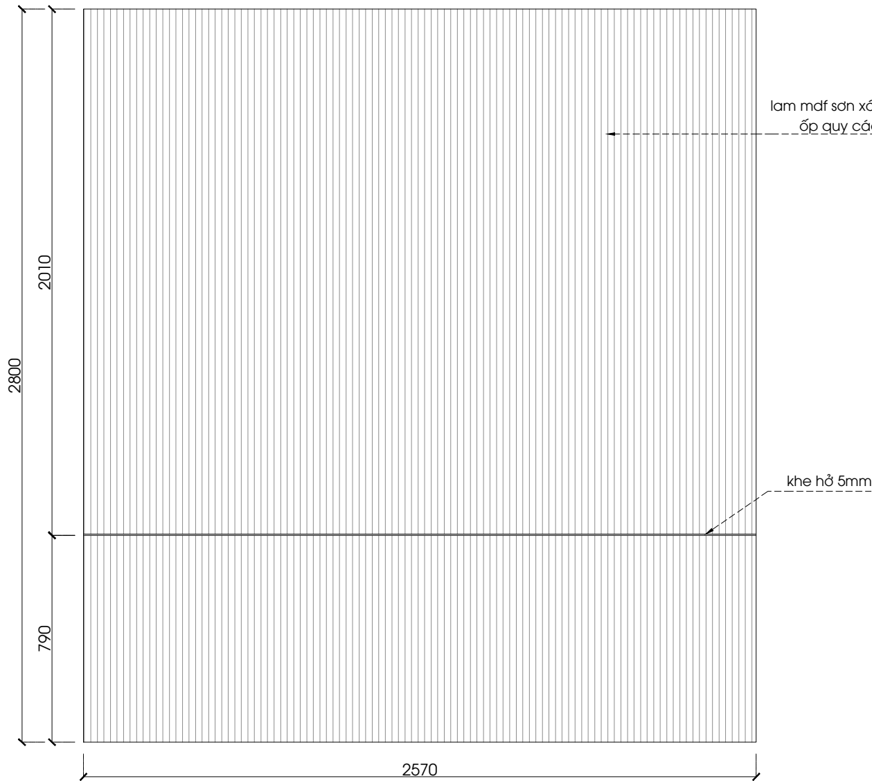
MẶT ĐỨNG 1 PM-02 1:20 @A3
