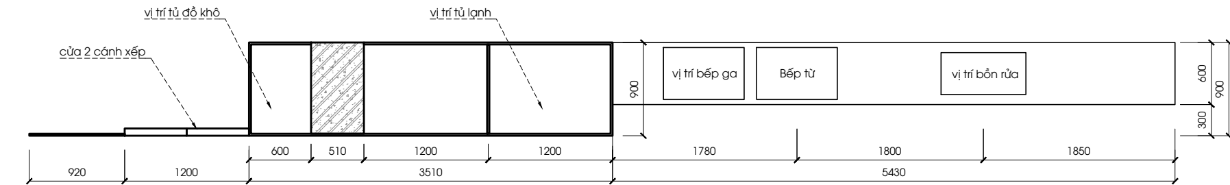
MẶT BẰNG HỆ TỦ BẾP
