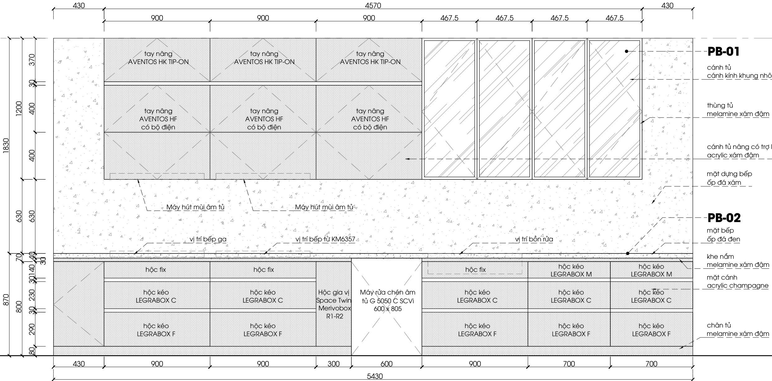
PB-01 & PB-02 - MẶT ĐỨNG 1:20 @ A3
