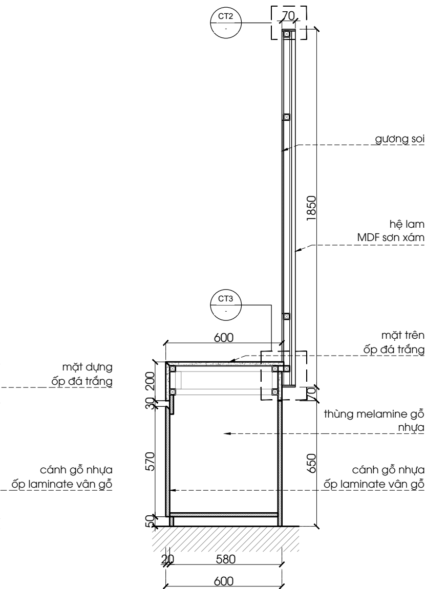
MẶT CẮT 1
