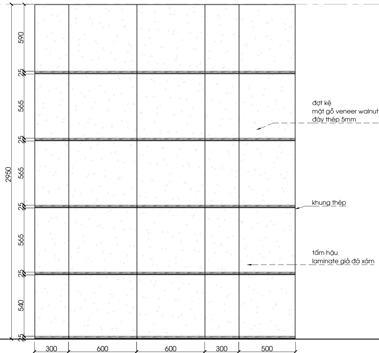
PP-01 - MẶT ĐỨNG
