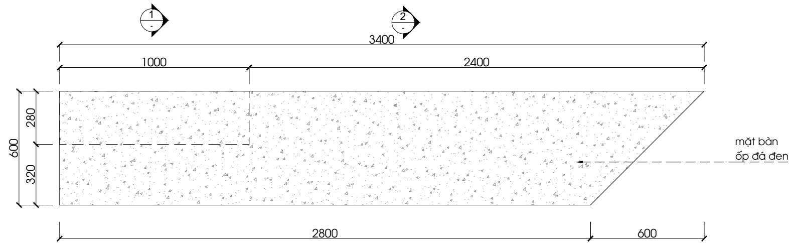
PN1- 02- MẶT BẰNG 1:20 @ A3
