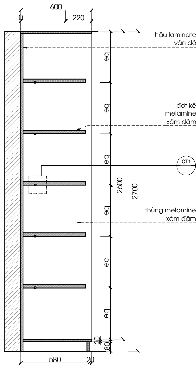
MẶT CẮT 1 1:20 @A3
