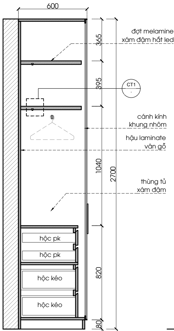
MẶT CẮT 2 1:20 @A3
