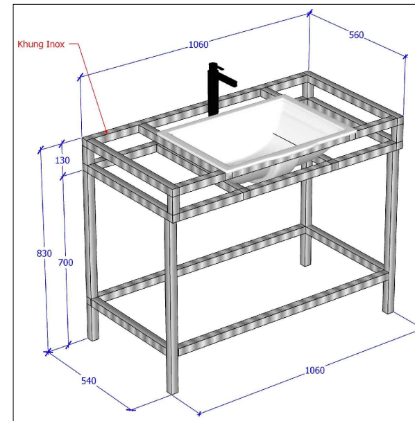
PN1-07 - PHỐI CẢNH KHUNG INOX
