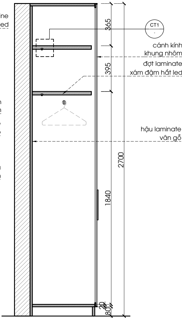
MẶT CẮT 3 1:20 @A3
