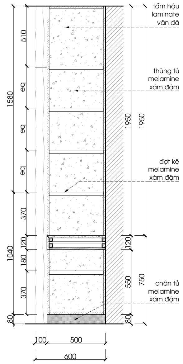
MẶT CẮT 5 1:20 @A3
