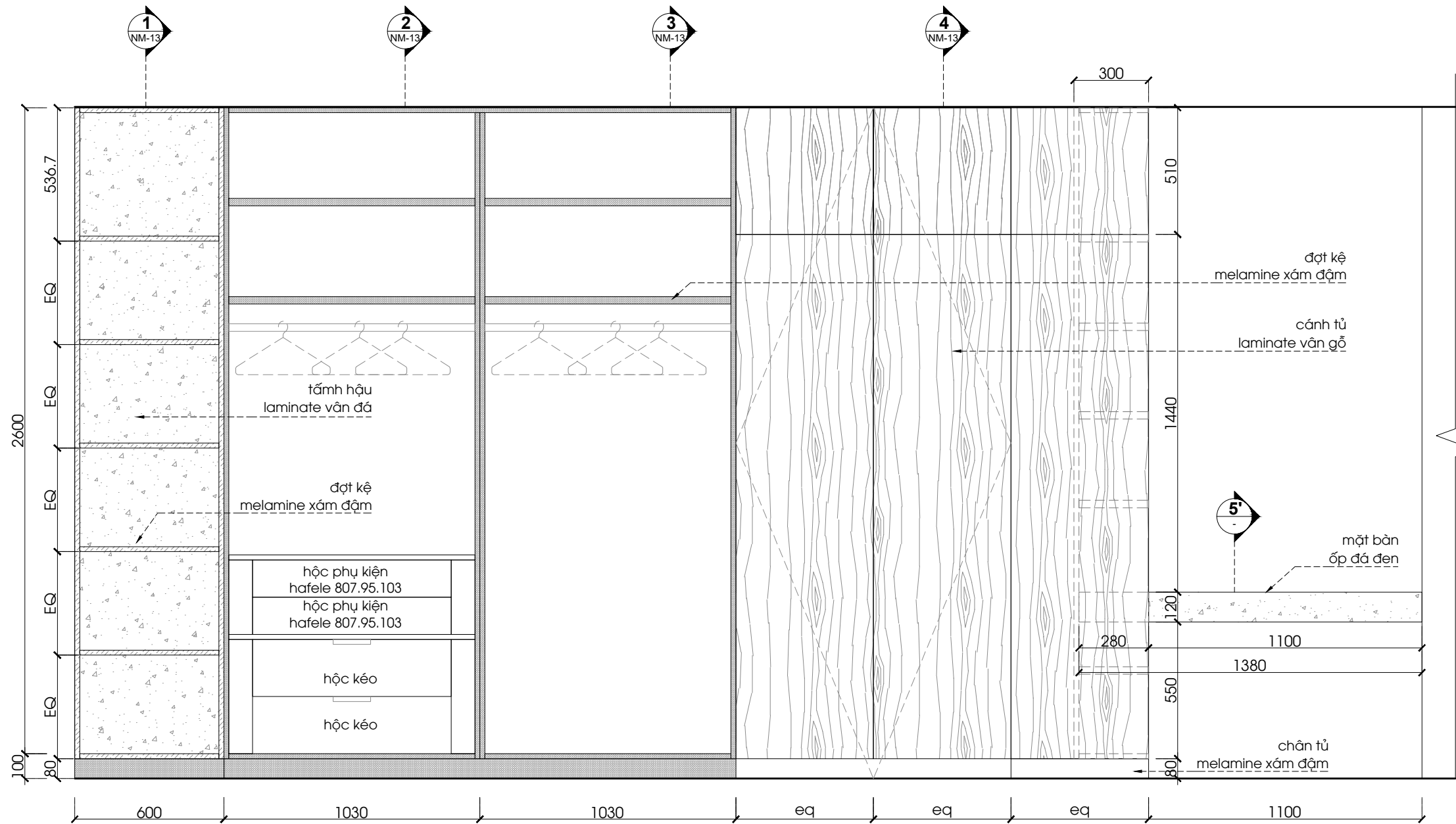
MẶT ĐỪNG PM-08,09,10 1:20 @A3
