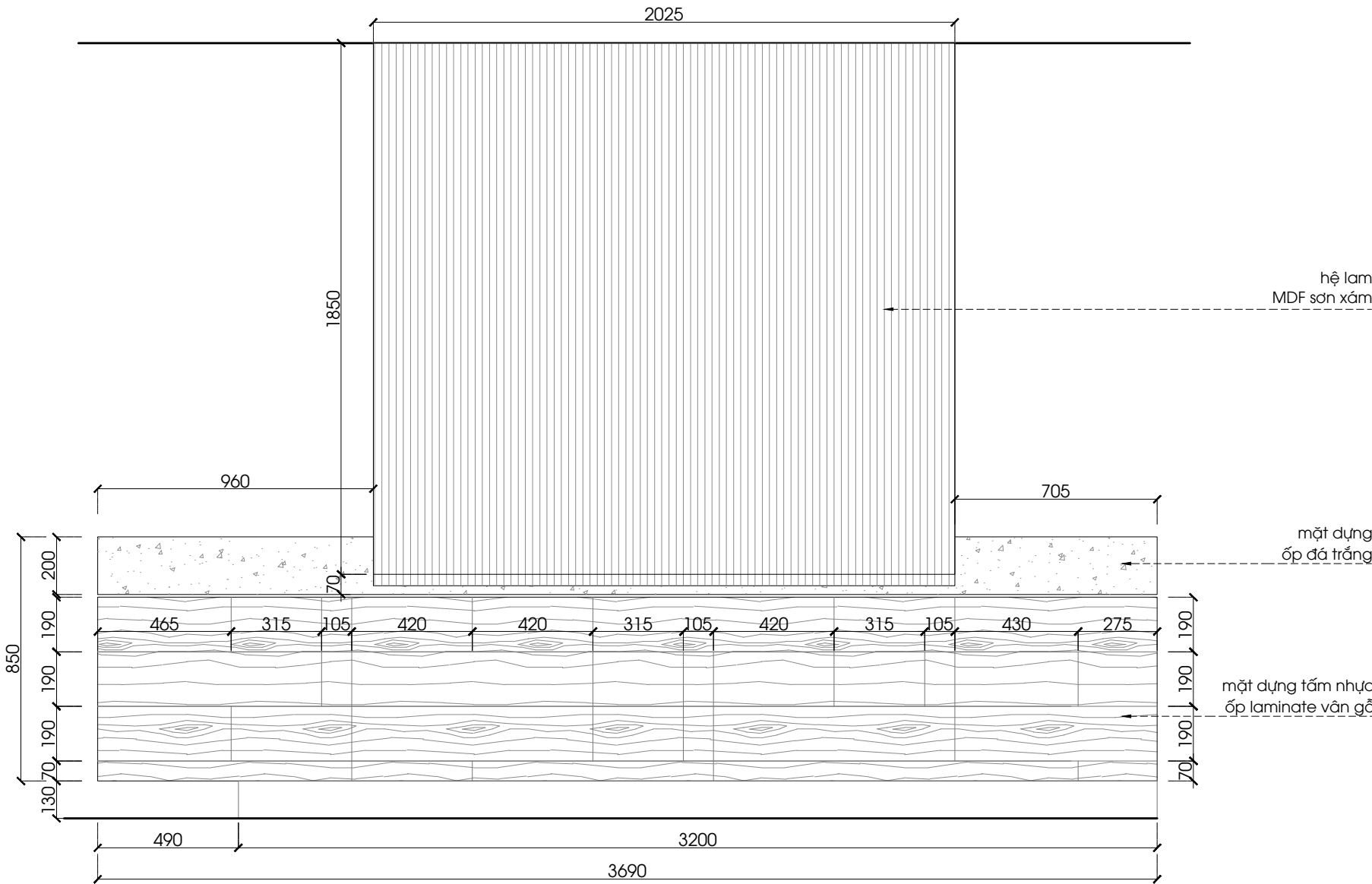
MẶT ĐỨNG 3 PM-12 1:20 @A3
