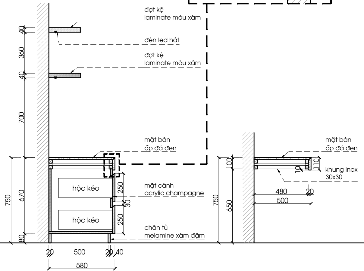
PN1- 02- MẶT CẮT 1 1:20 @ A3
