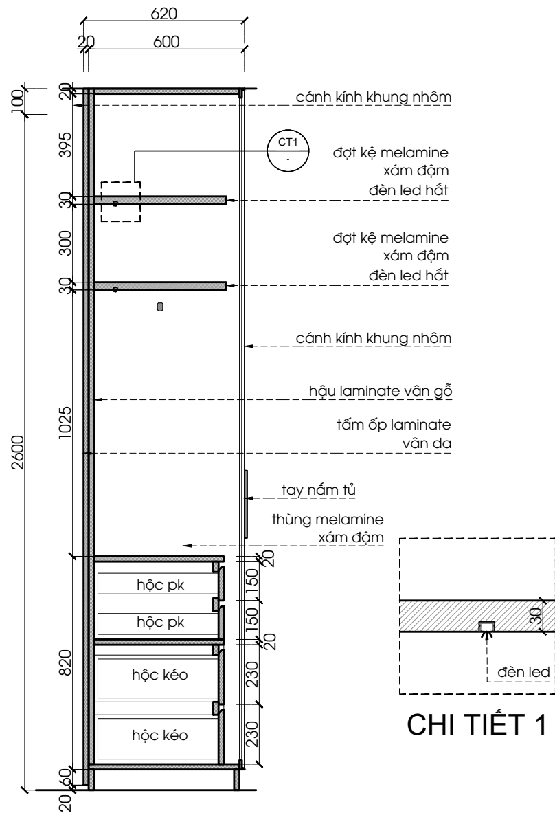
MẶT CẮT 1 1:20 @A3
