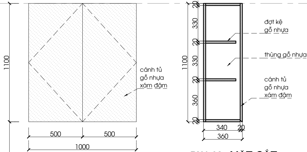
PN1-08 - MẶT CẮT 1:20 @ A3
