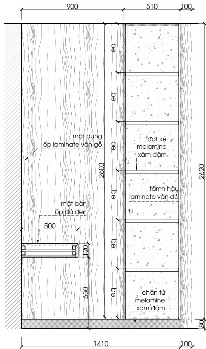
MẶT CẮT 5' 1:20 @A3
