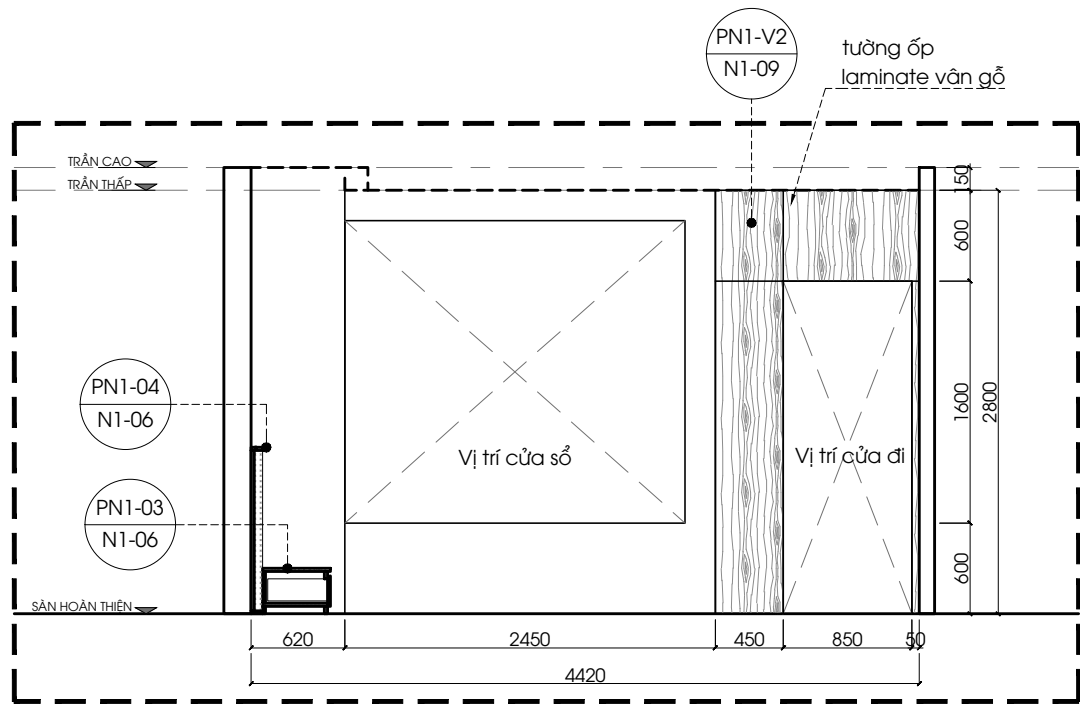
PN1 MẶT ĐỨNG 1
