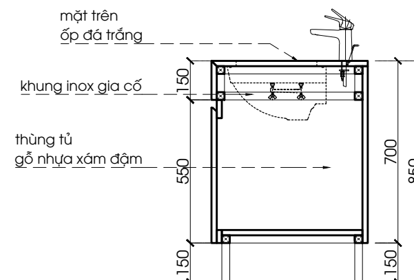
PN1-07 - MẶT CẮT 1:20 @ A3
