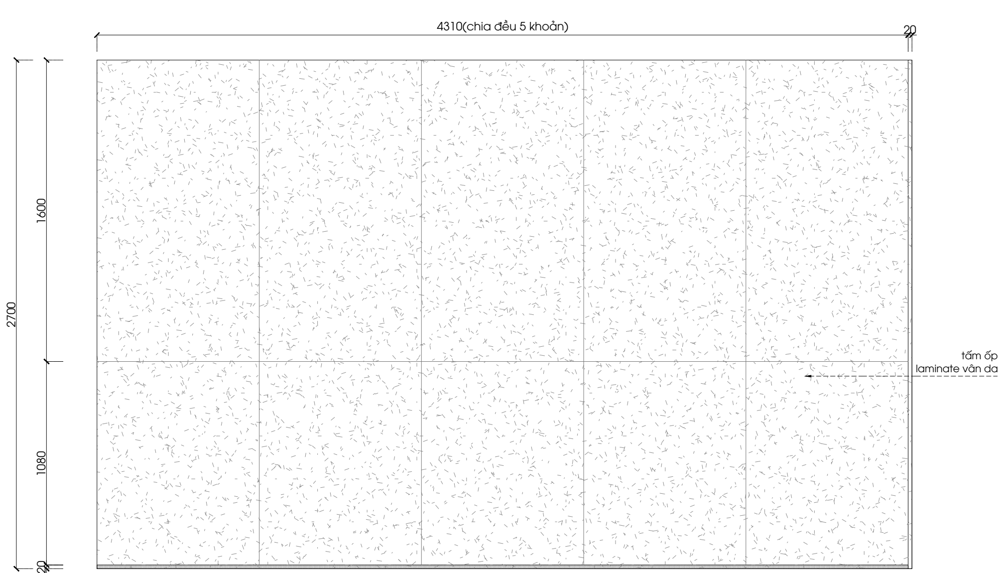
MẶT ĐỪNG PM-V6 1:20 @A3
