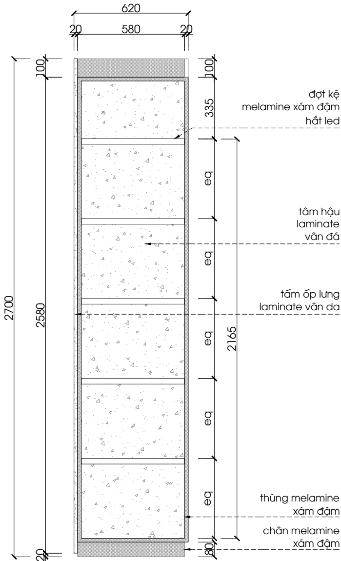
MẶT ĐỪNG PM-06 1:20 @A3
