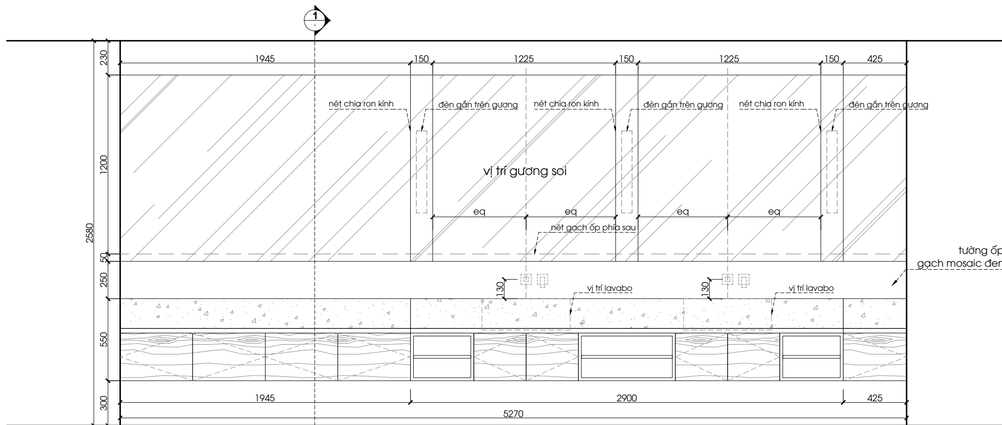
WC-01 MẶT ĐỨNG
