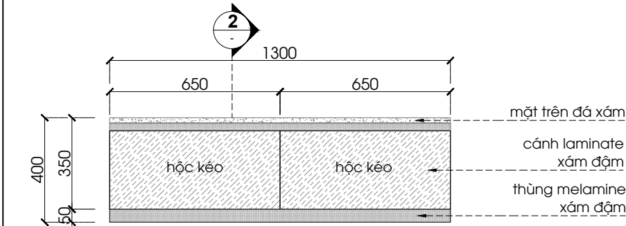
MẶT ĐỪNG PM-04 1:20 @A3
