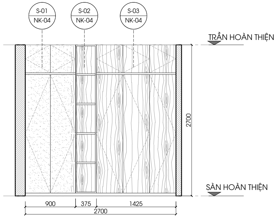
MẶT ĐỨNG 2 1:40 @A3
