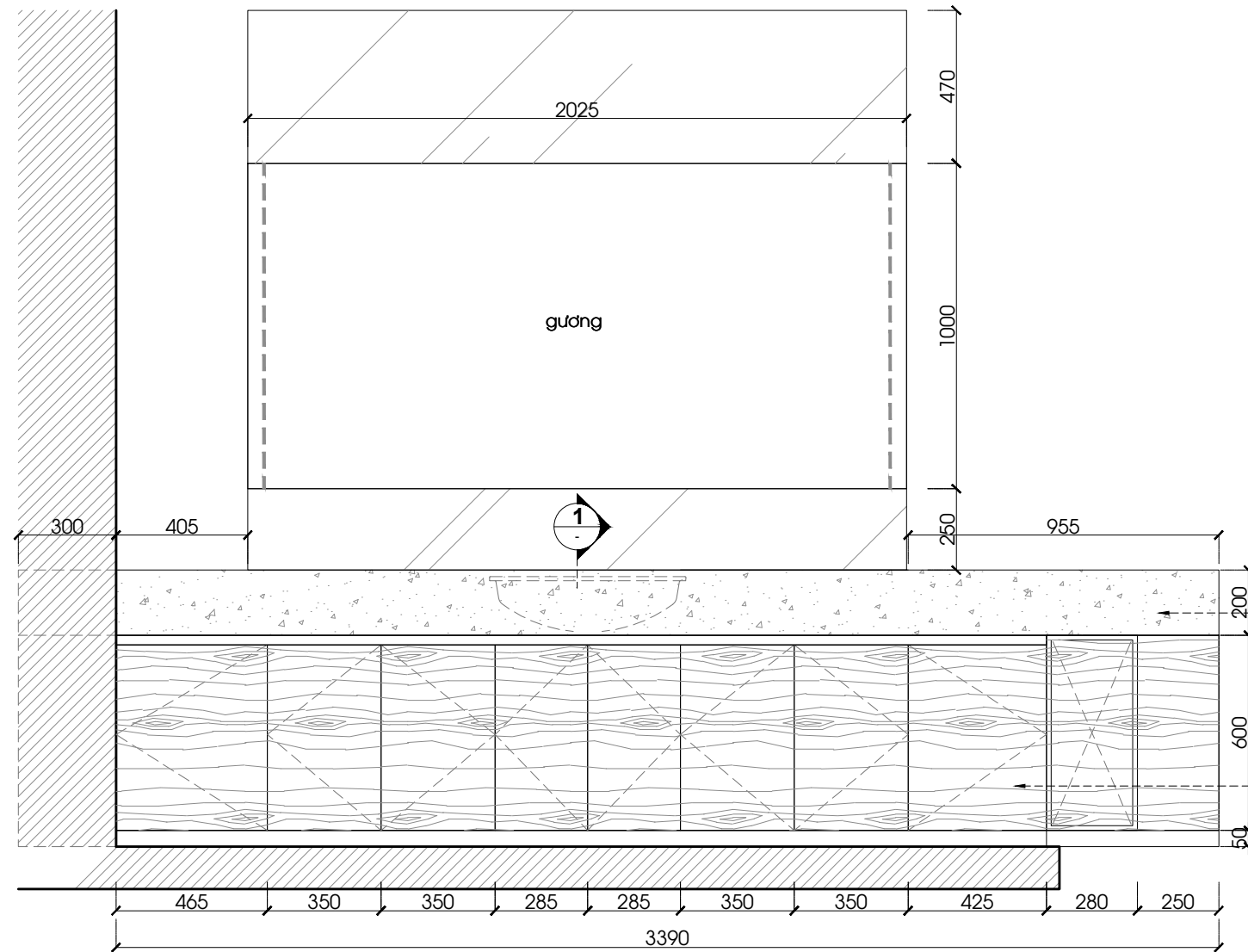
MẶT ĐỪNG 1 PM-12
