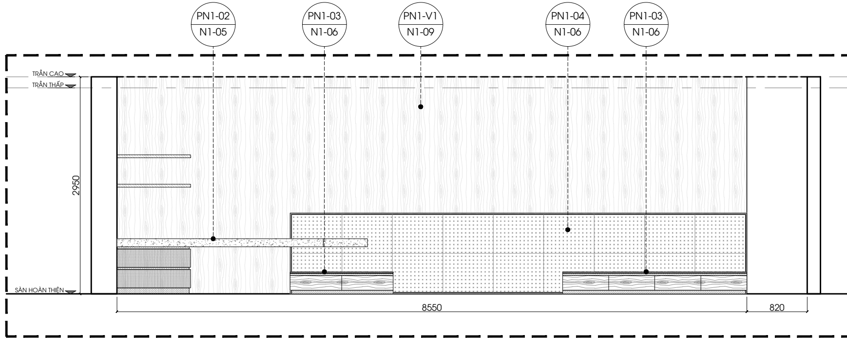
PN1 MẶT ĐỨNG 4
