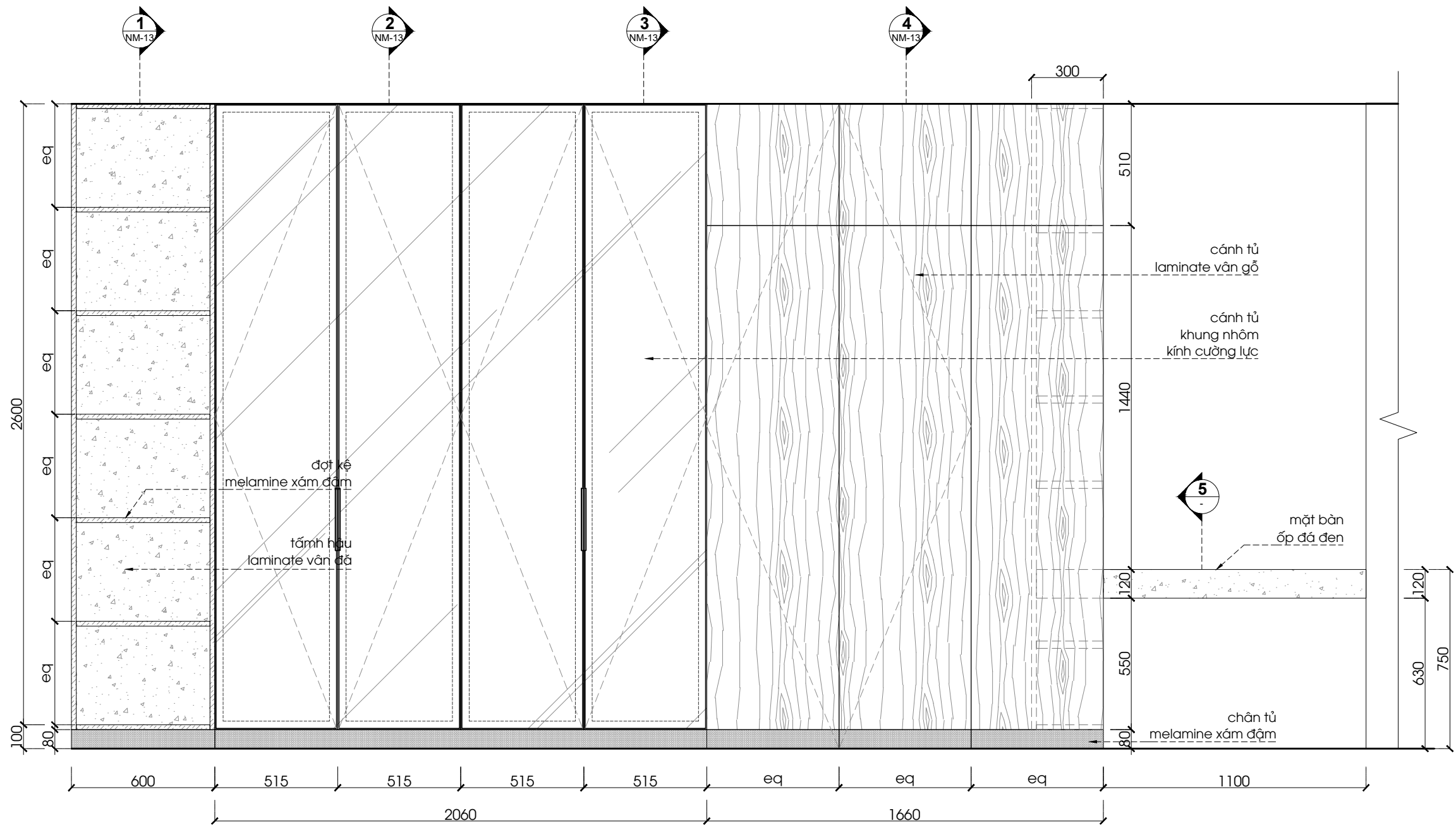
MẶT ĐỨNG PM-08,09,10 1:20 @A3
