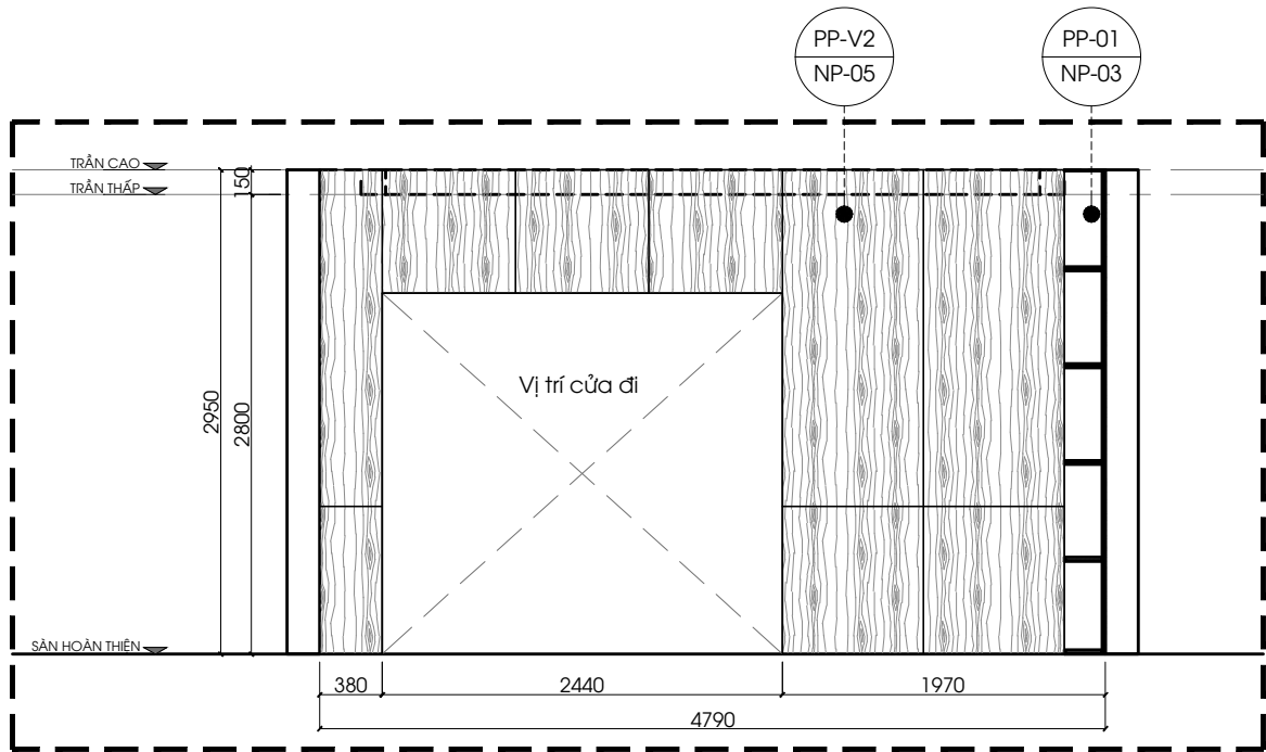
PN1 MẶT ĐỨNG 1 - 1:50 @ A3
