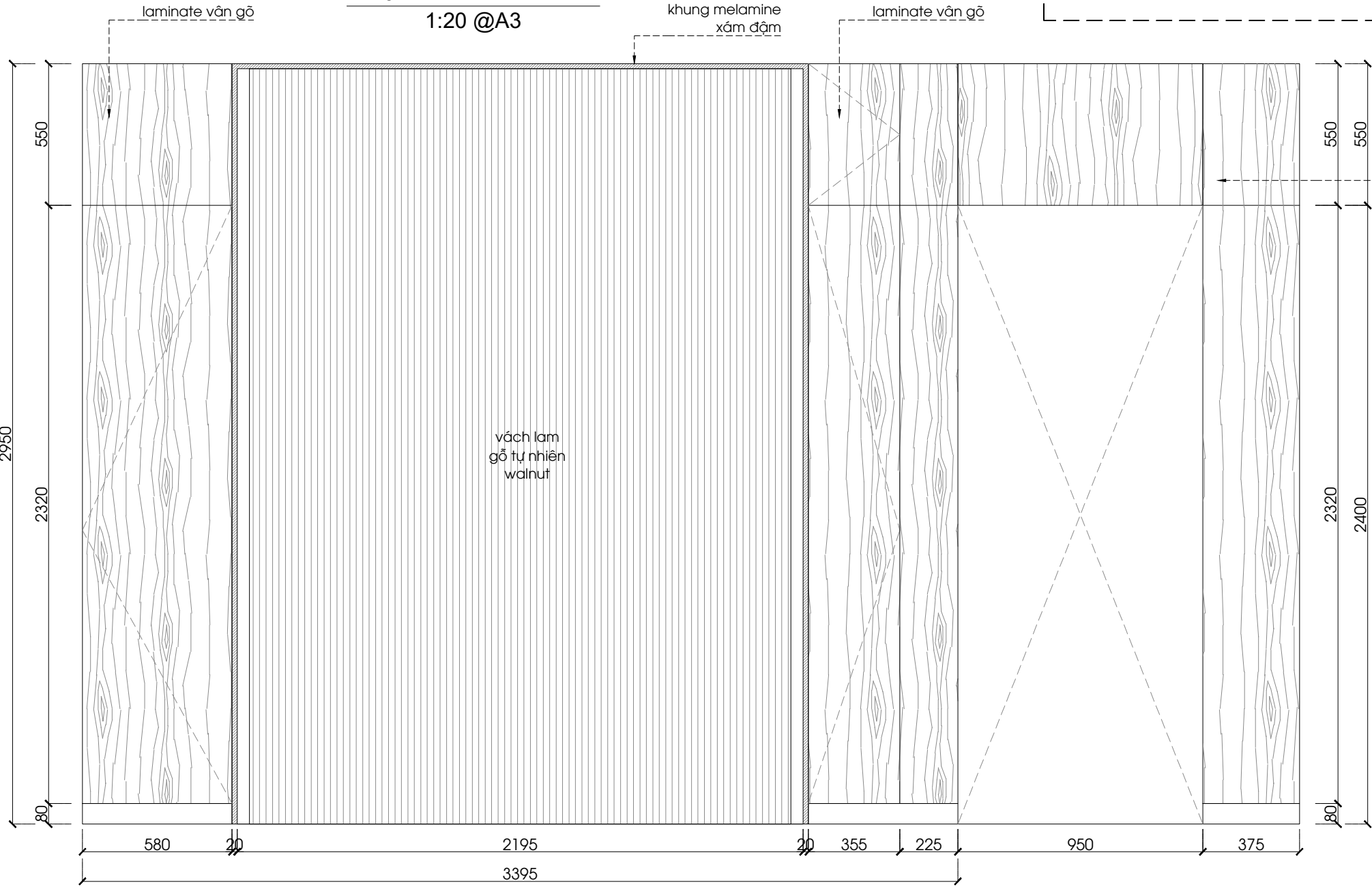
MẶT ĐỪNG PK-03 1:20 @A3
