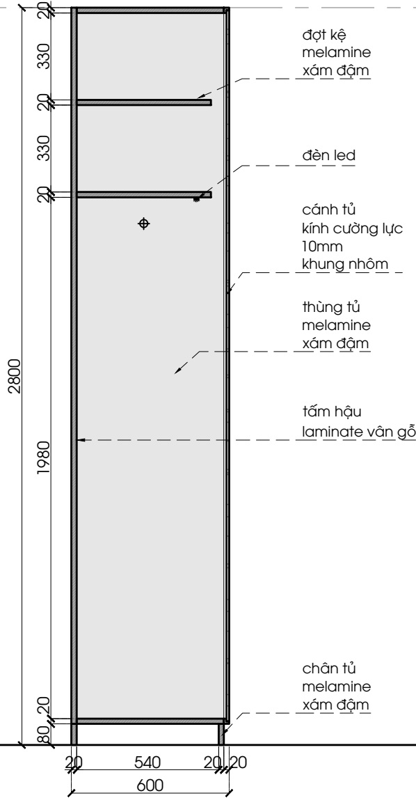
PN1-01- MẶT CẮT 1 1:20 @ A3
