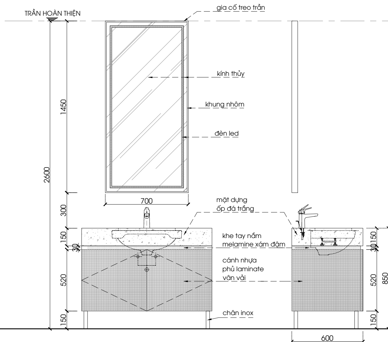
PN1-07 - MẶT ĐỨNG 1:20 @ A3
