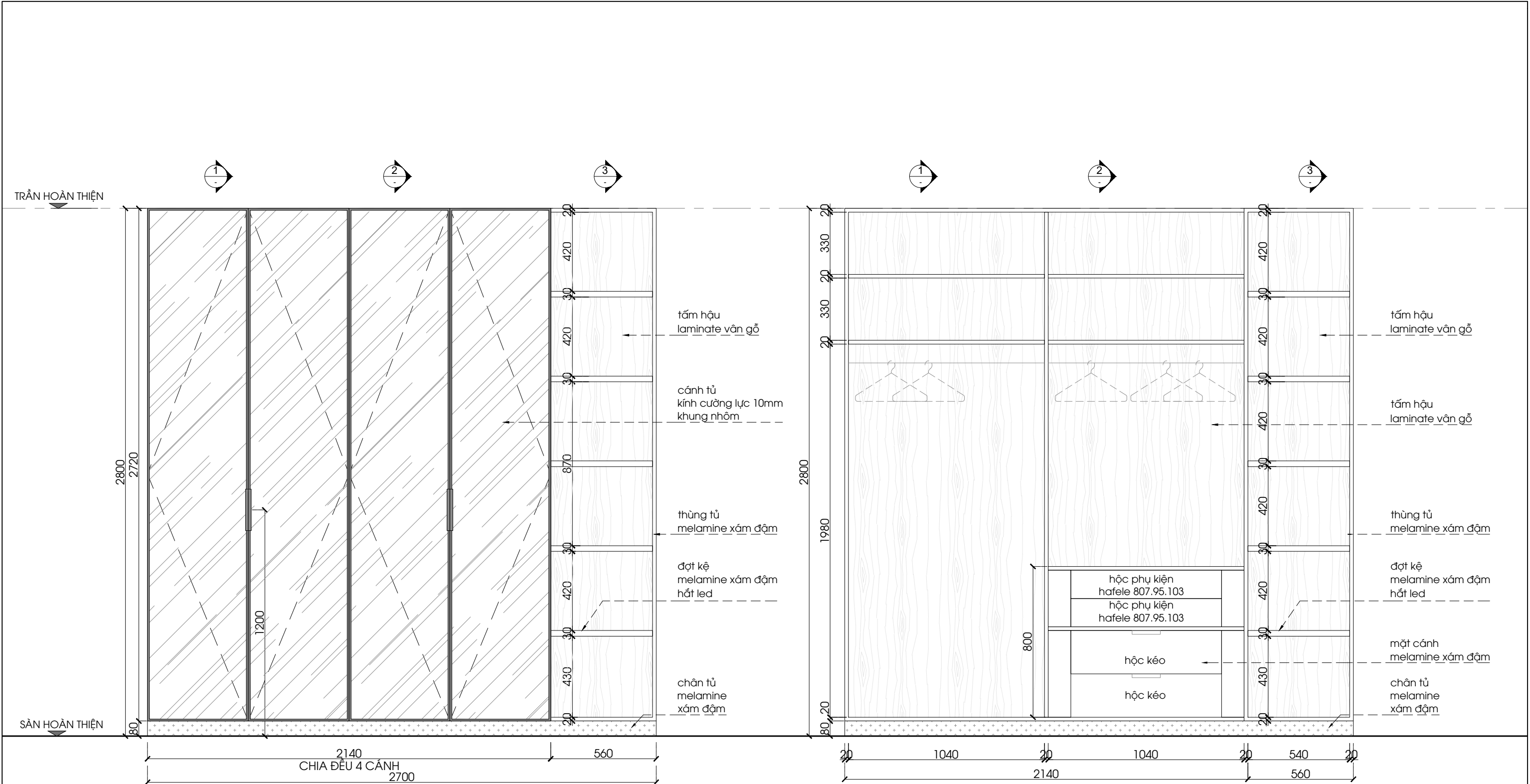
PN1- 01- MẶT ĐỪNG
