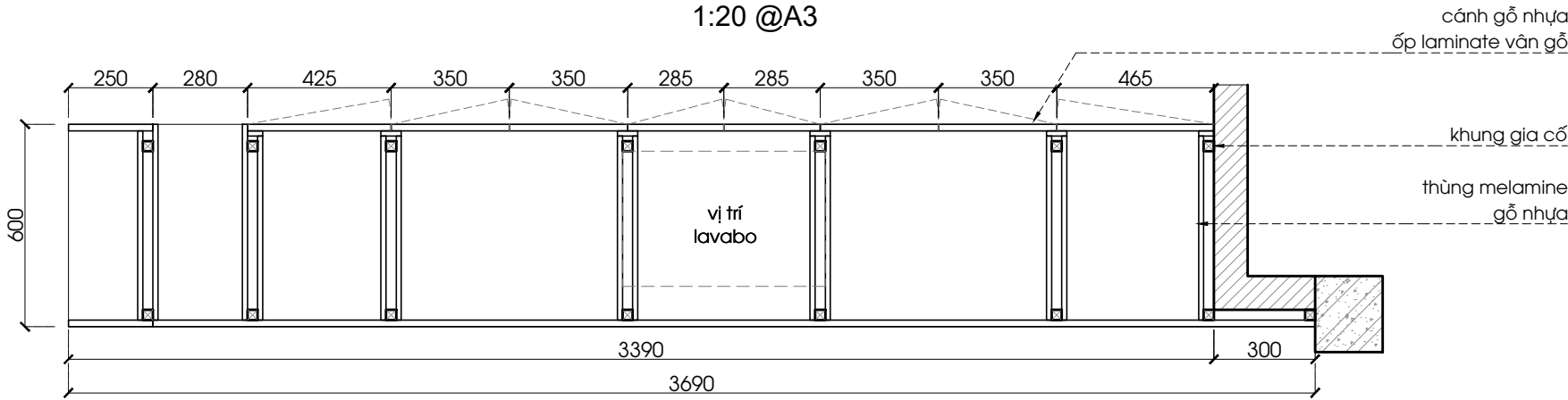
MẶT BẰNG THÙNG TỦ PM-12 1:20 @A3
