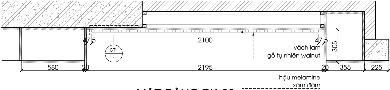
MẶT BẰNG PK-03 1:20 @A3
