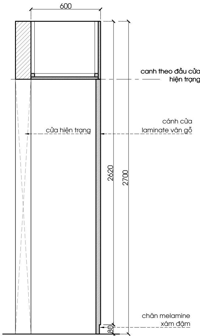
MẶT CẮT 4 1:20 @A3
