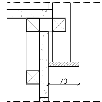
CHI TIẾT 3
