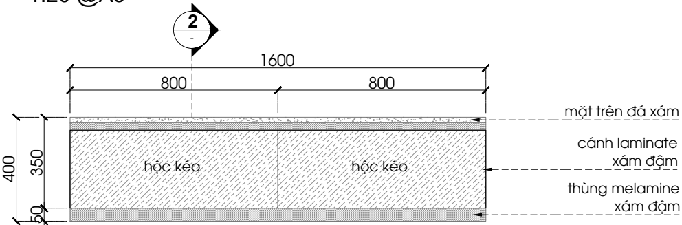
MẶT ĐỪNG PM-05 1:20 @A3
