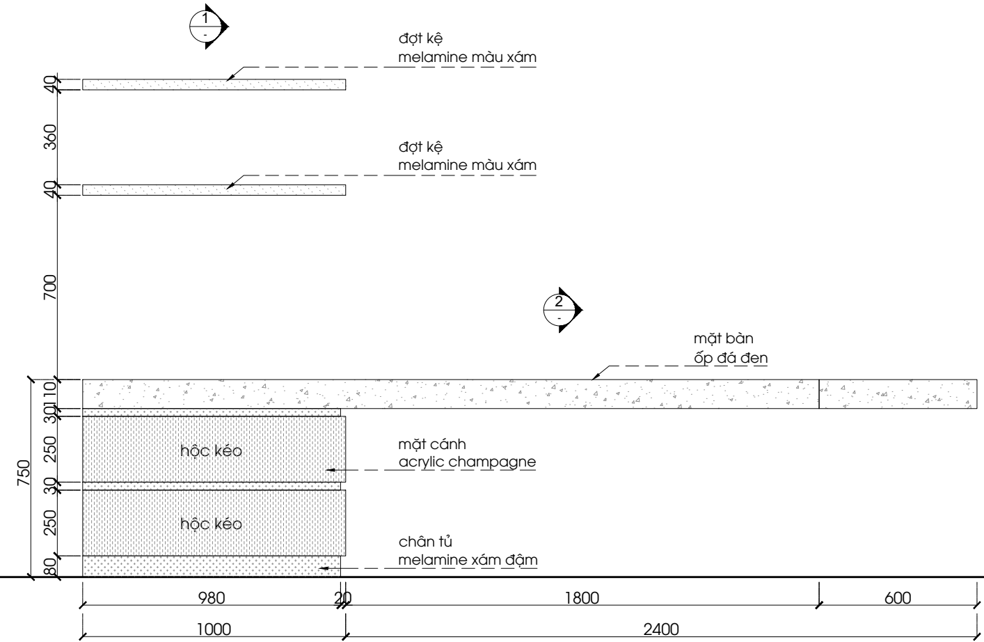
PN1- 02- MẶT ĐỨNG 1:20 @ A3
